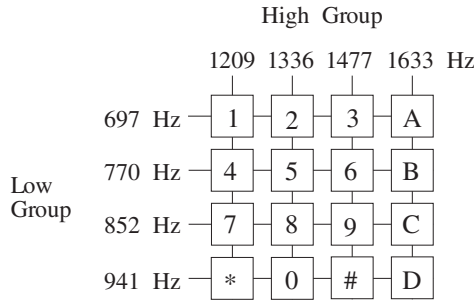
Fig. 8.1.3 DTMF keypad.
